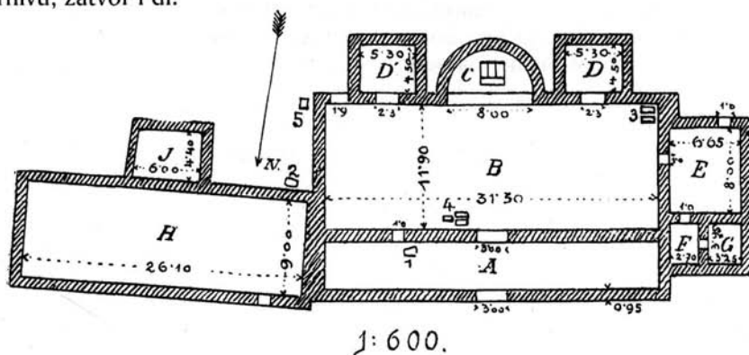
Sl. 5. Tlocrt gradske vijećnice (Gradina – Domavia)
