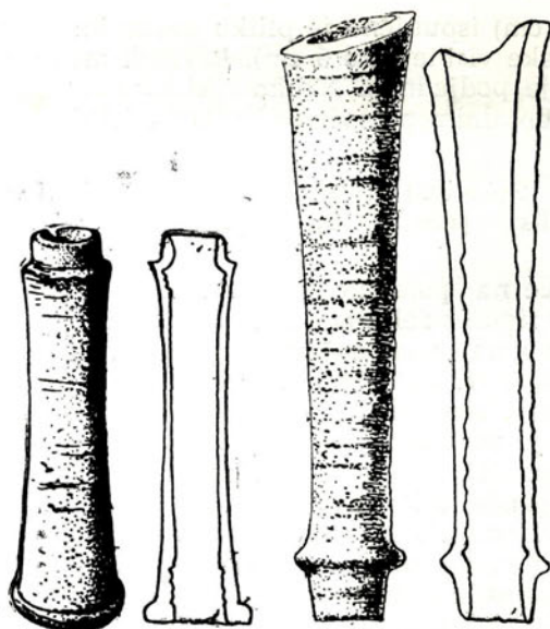
Sl. 6 — Keramičke cijevi od vodovoda iz Rogatice (1 : 4)
