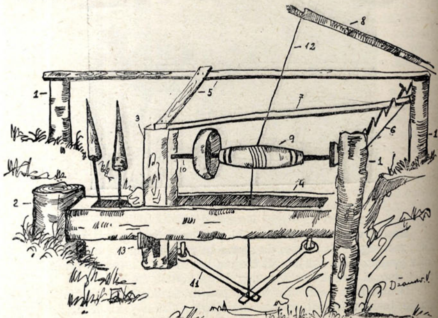
Crtež 1 — »muški terdžaj«. 1. paru, 2. furka (sova), 3. zeoru, 4. doaga, 5. puntija (čuprija), 6. Krjasta, 7. citorju, 8. pržna (srg), 9. valu (vreteno), 10. šiljak, 11. klkatorilji, 12. kaiš, 13. pana.
