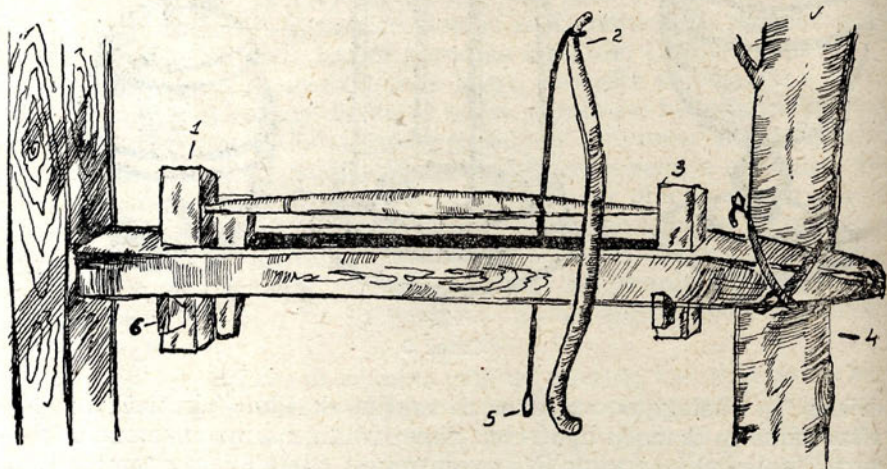
Crtež 7 — »ženski terdžaj«. 1. zeoru, 2. arkušu (gudalo), 3. kljimpšu, 4. bcu (štap), 5. deđetaru (omča od kože), 6. pana (zaglavak).
