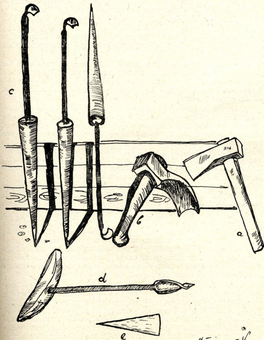
Crtež 8 — čančarski alat: a) sikira, b) tesla, c) dubač, d) svrdlo, e) gruka.
