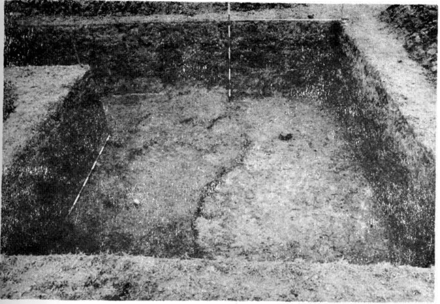
Sl. 24 Lok. »Korića Han«, sonda VIII
