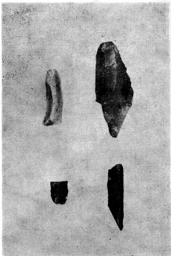
Sl. 78. Kameni odbici i nukleusi
