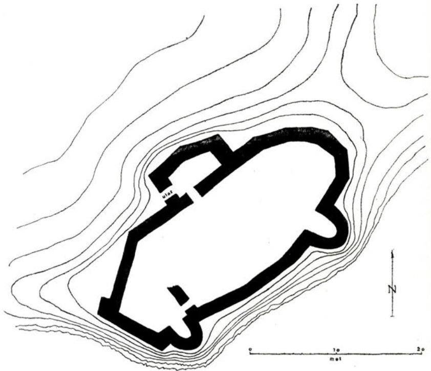
Sl. 1. — Grad Sokol — tlocrt
